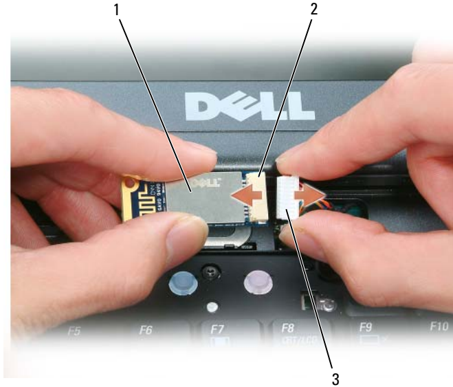
1 插卡 2 插卡连接器 3 电缆连接器
